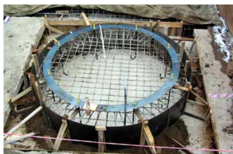
Betonáž základů nádrže.
